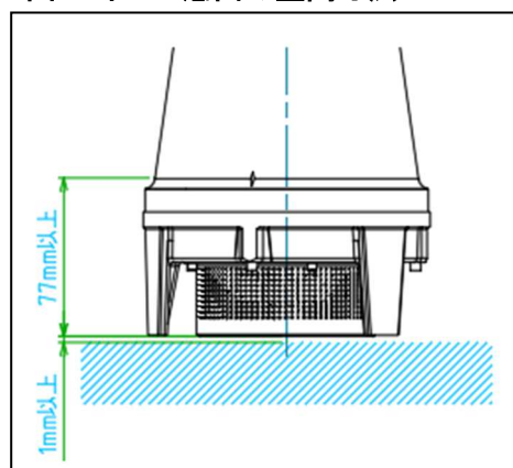
図4. ポンプ底面の空間寸法
