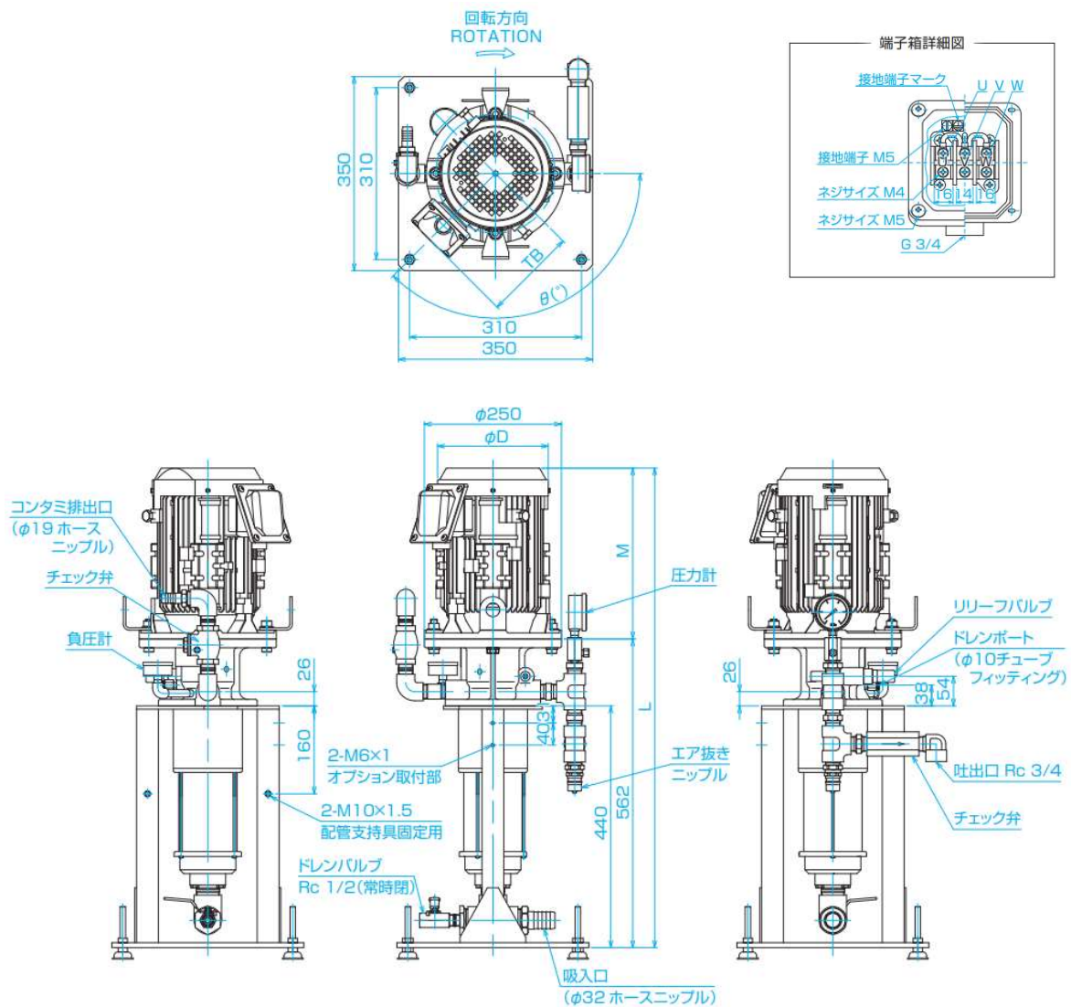
図 2. ポンプ外観寸法
