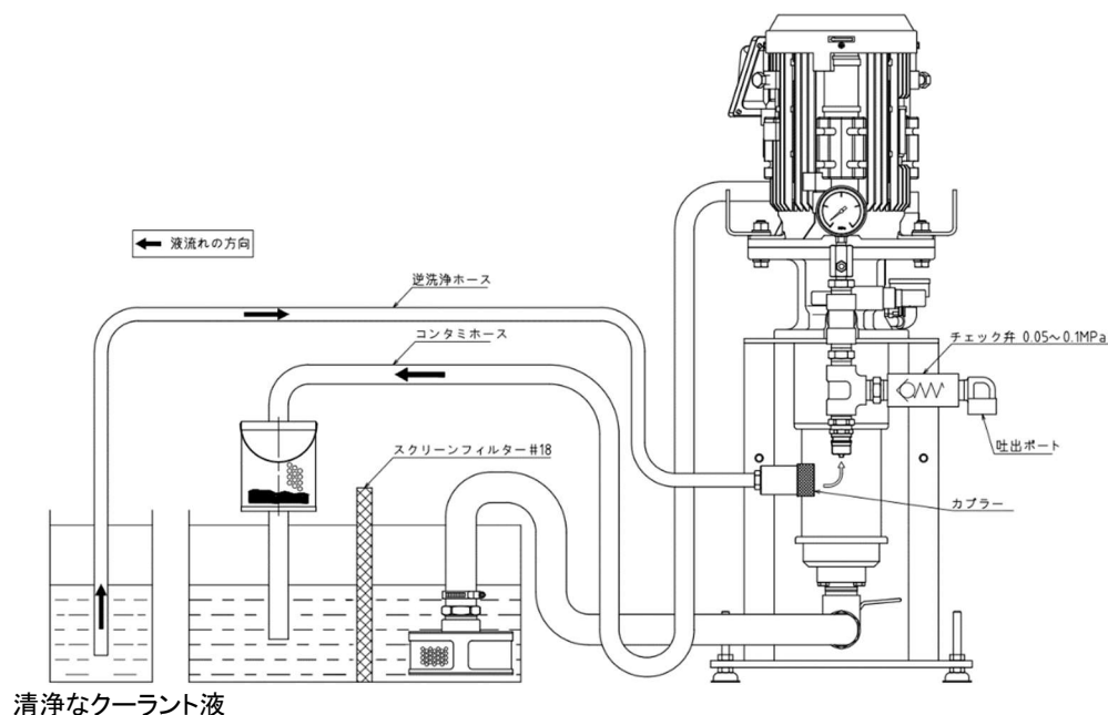
図 10. 逆洗浄推奨設置図
