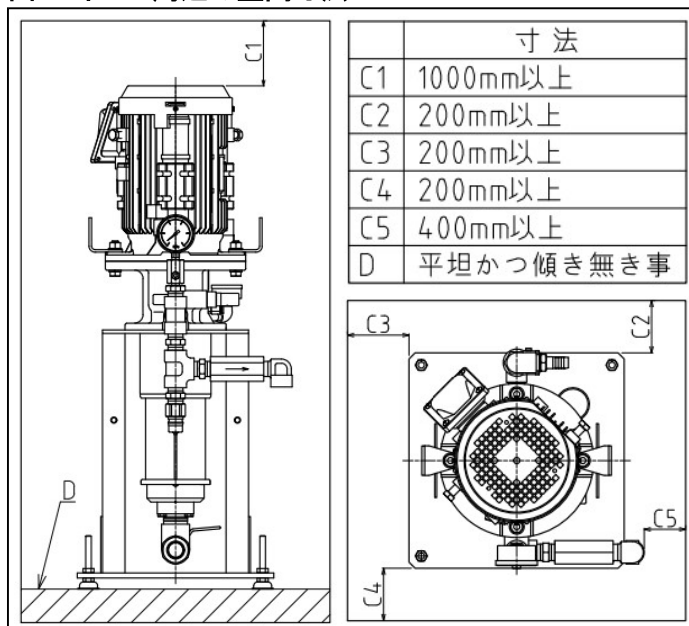
図 4. ポンプ周辺の空間寸法
