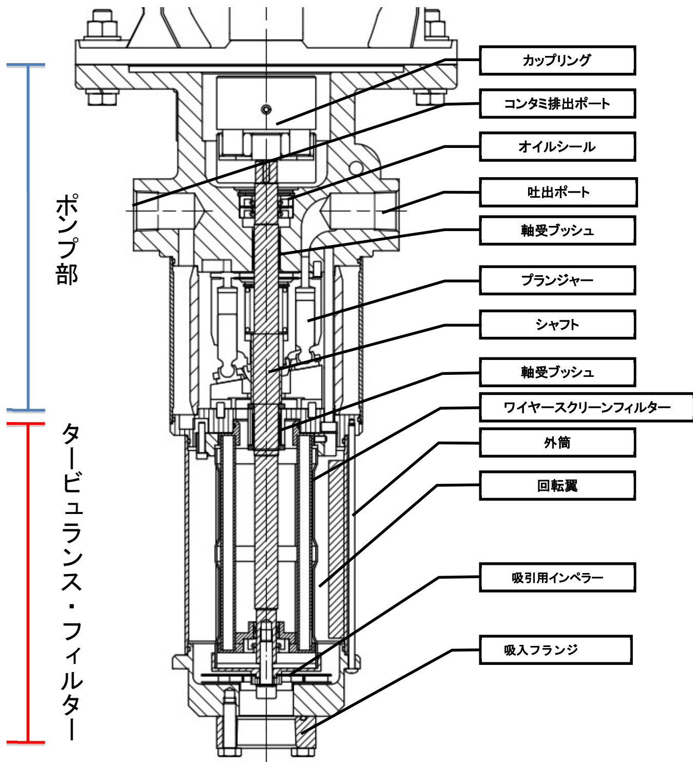
図 9. ポンプ各部名称
