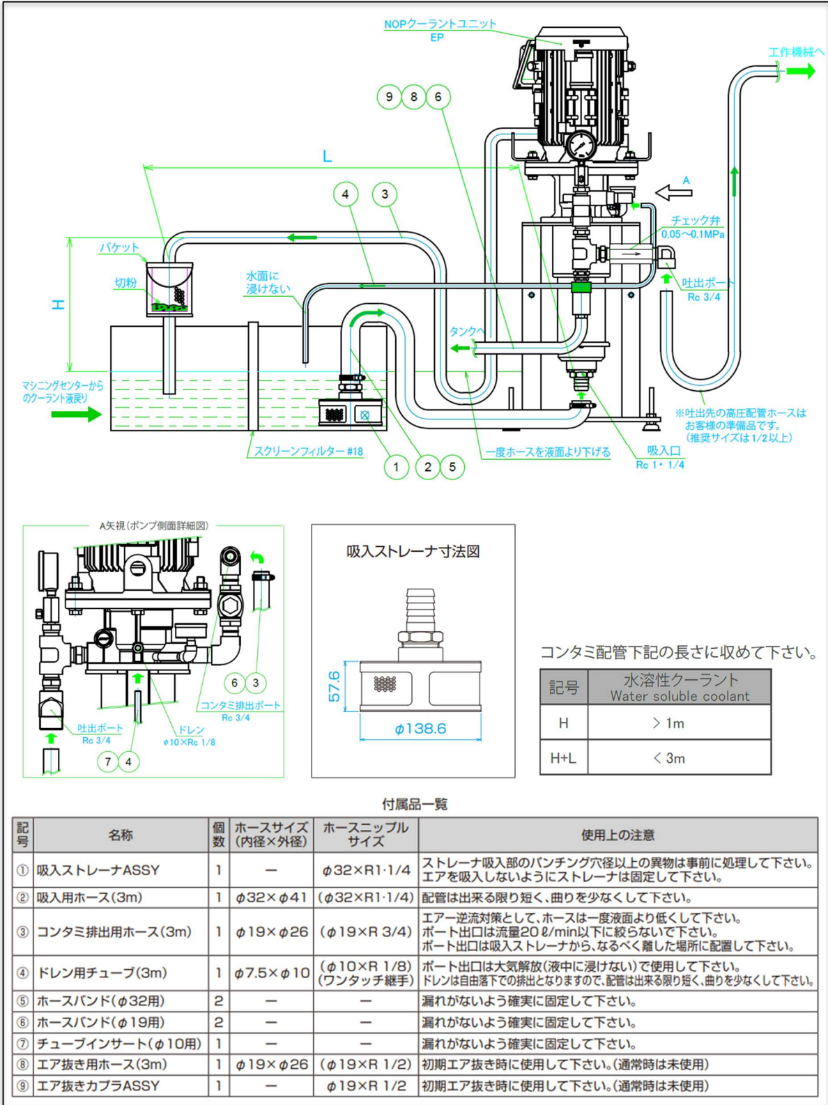
図 7. 設置要領図
