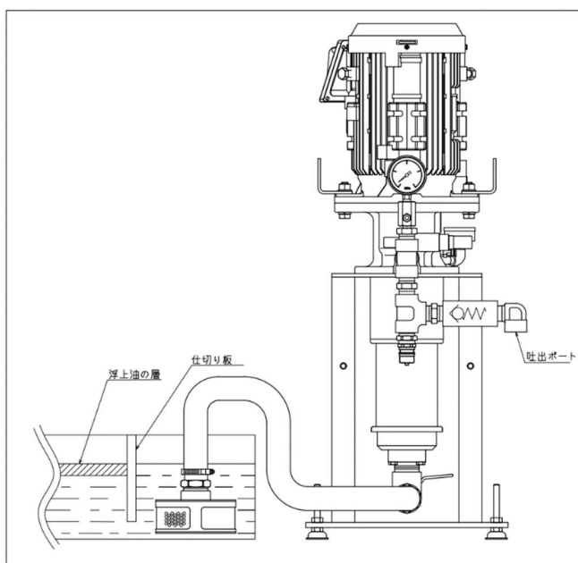
図 6. 浮上油対策の参考図
