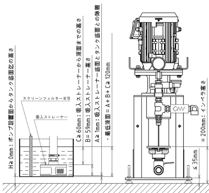
図 5. 吸入ストレーナー位置と最低液面
