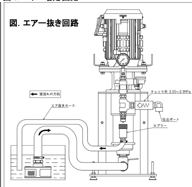
図 3. エア抜き回路
