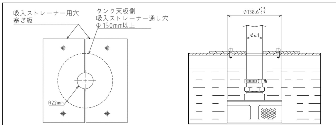
図 1. 吸入ストレーナー取付け穴寸法
