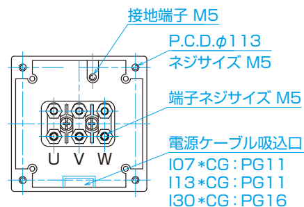
端子箱詳細図
