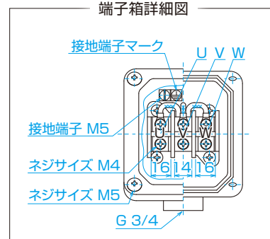
端子箱詳細図
