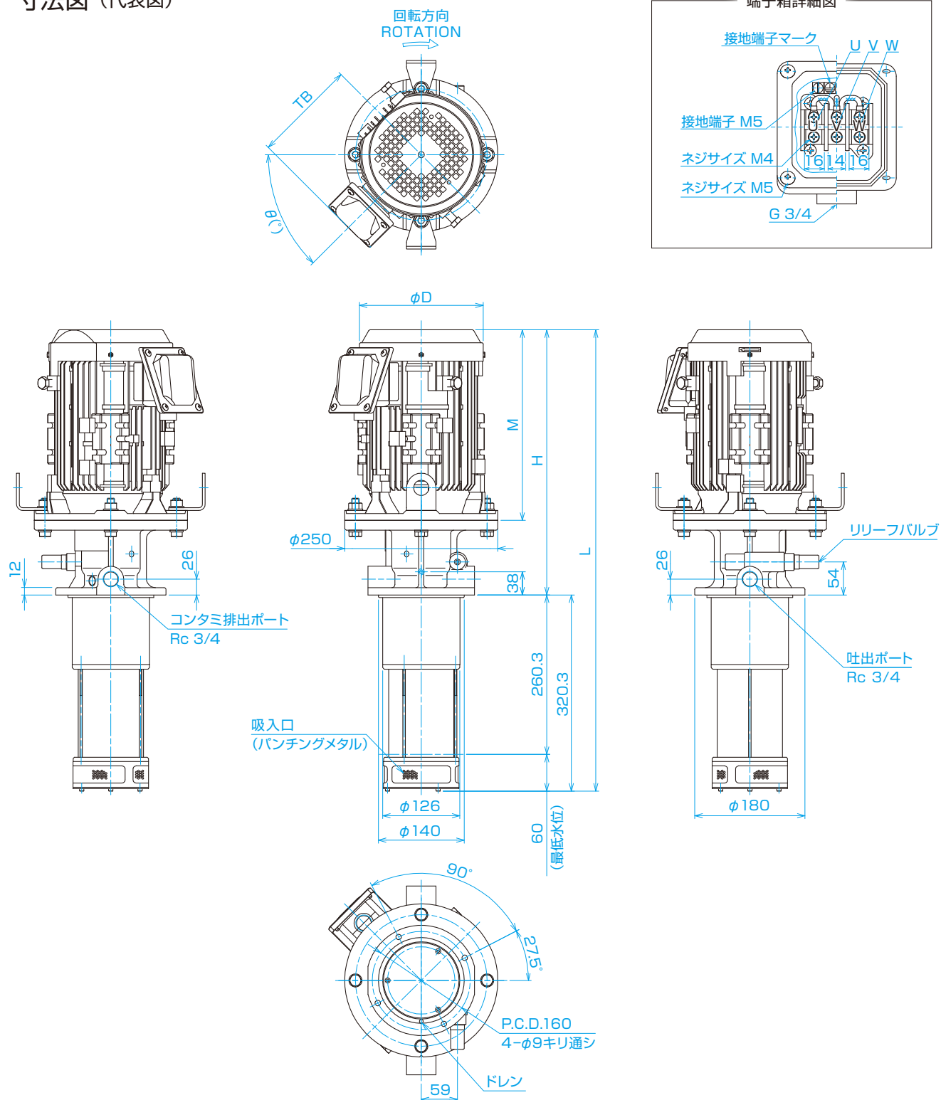
寸法図 (代表図)
