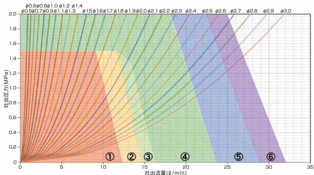
— NOPフィルターポンプYTH-ES ツール2穴用 吐出範囲グラフ —
